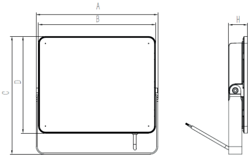
Dimensional Drawing / طراحی بعدی
