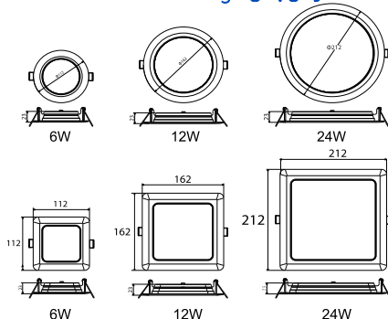
Dimensional Drawing / طراحی بعدی
