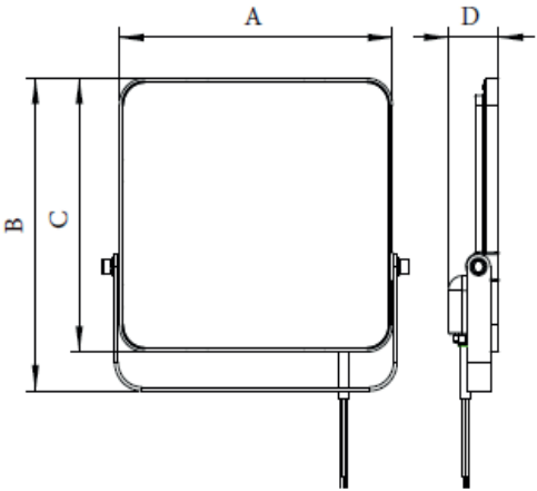
Dimensional Drawing / طراحی بعدی
