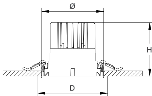
طراحی بعدی / Dimensional Drawing
