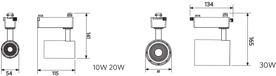
طراحی بعدی / Dimensional Drawing
