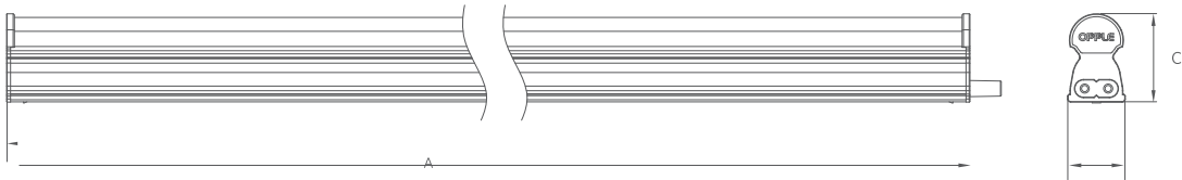
طراحی بعدی / Dimensional Drawing
