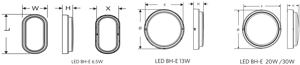
Dimensional Drawing / طراحی بعدی
