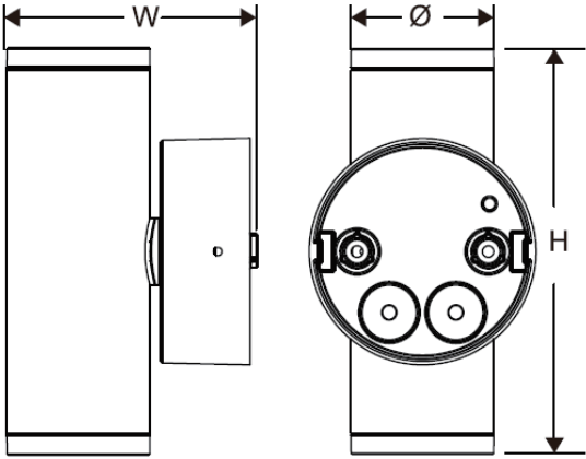
طراحی بعدی / Dimensional Drawing
