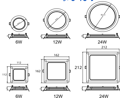
Dimensional Drawing / طراحی بعدی
