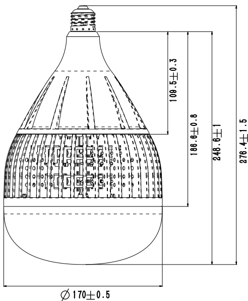
طراحی بعدی / Dimensional Drawing
