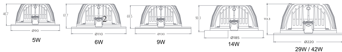
Dimensional Drawing / طراحی بعدی
