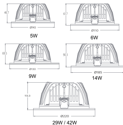
Dimensional Drawing / طراحی بعدی
